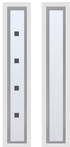
Sophie Pièces métalliques en applique (en option) Décor fusion V8SPA3 (en option) H max: 2383 mm - H min: 1988 mm L max: 1113 mm - L min: 877 mm Coef. Ud: 1,4
